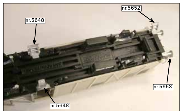
Foto 10: Gemonteerde trappetjes
