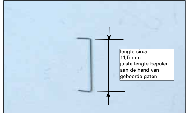
Foto 4: Gebogen handgrepen
