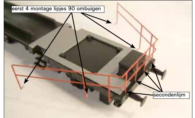
Foto 24: Plaatsen gebogen hekwerk
