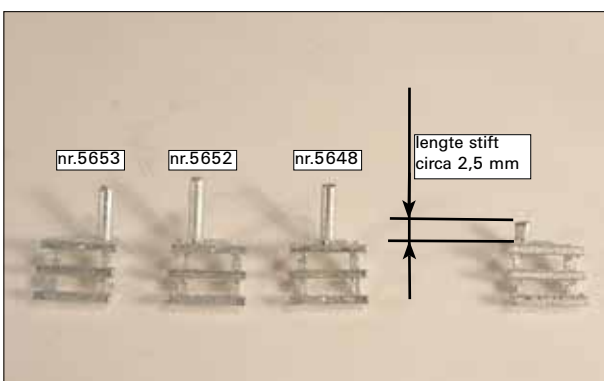
Foto 9: Trappetjes
