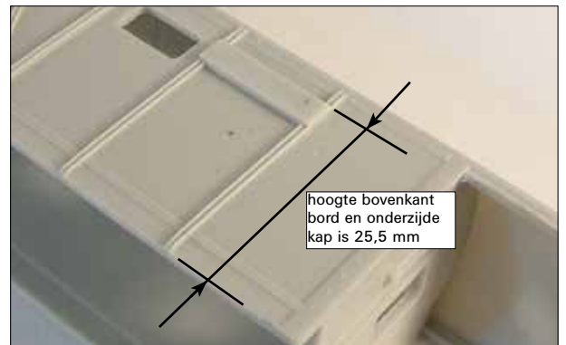
Foto 6: Positie Strukton bord
