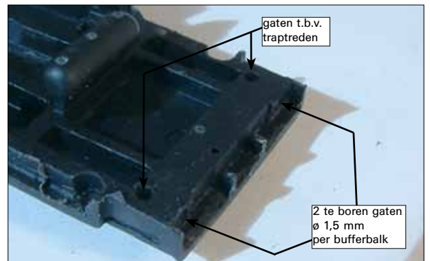
Foto 8: Bufferbalk
