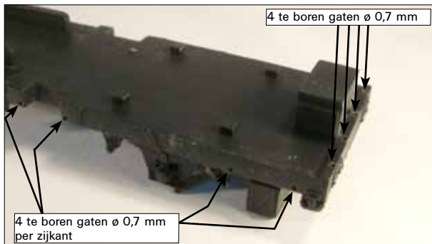
Foto 11: Te boren gaten t.b.v. hekwerk, ø 0,7 mm, 12 stuks totaal
