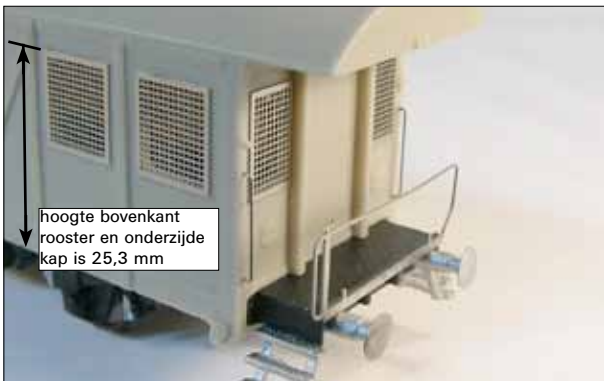
Foto 5: Gemonteerde handgrepen en bordeshek
